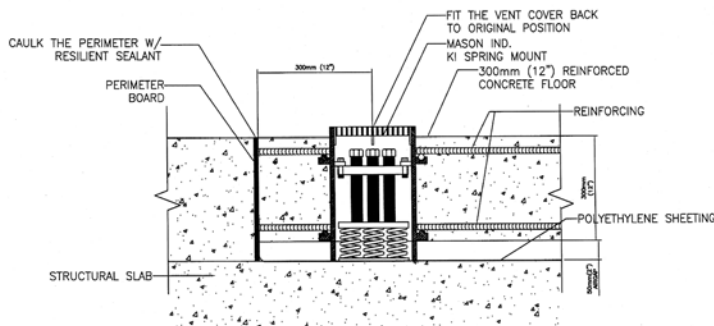
“MASON” KI 型自升式彈簧減震器裝置剖面圖
