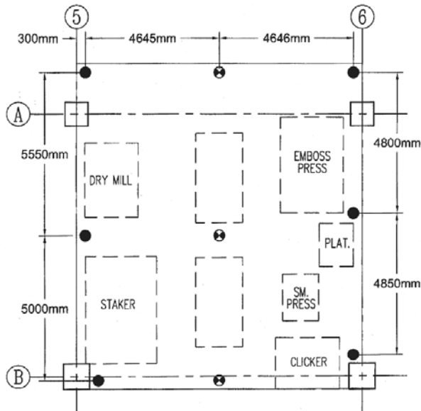
10 x11 米浮筑地板平面布置圖 (黑點為減震器位置)
