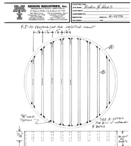
“MASON” KI 型彈簧減震器頂蓋設計圖
